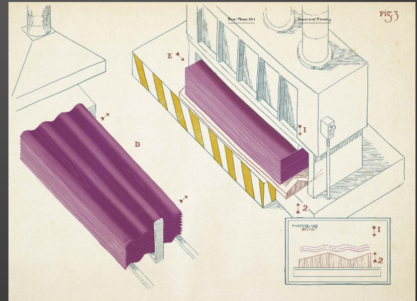
3-ia operacija - Presavimas
